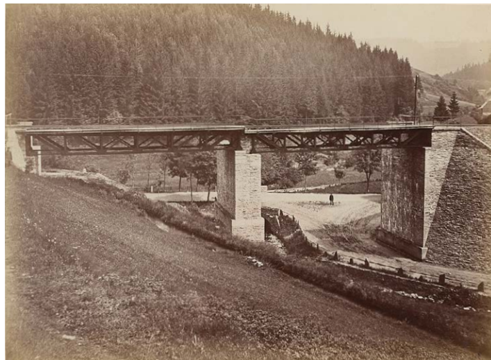
Eisenbahnbrücke über die Rote Pockau bei Rittersberg
